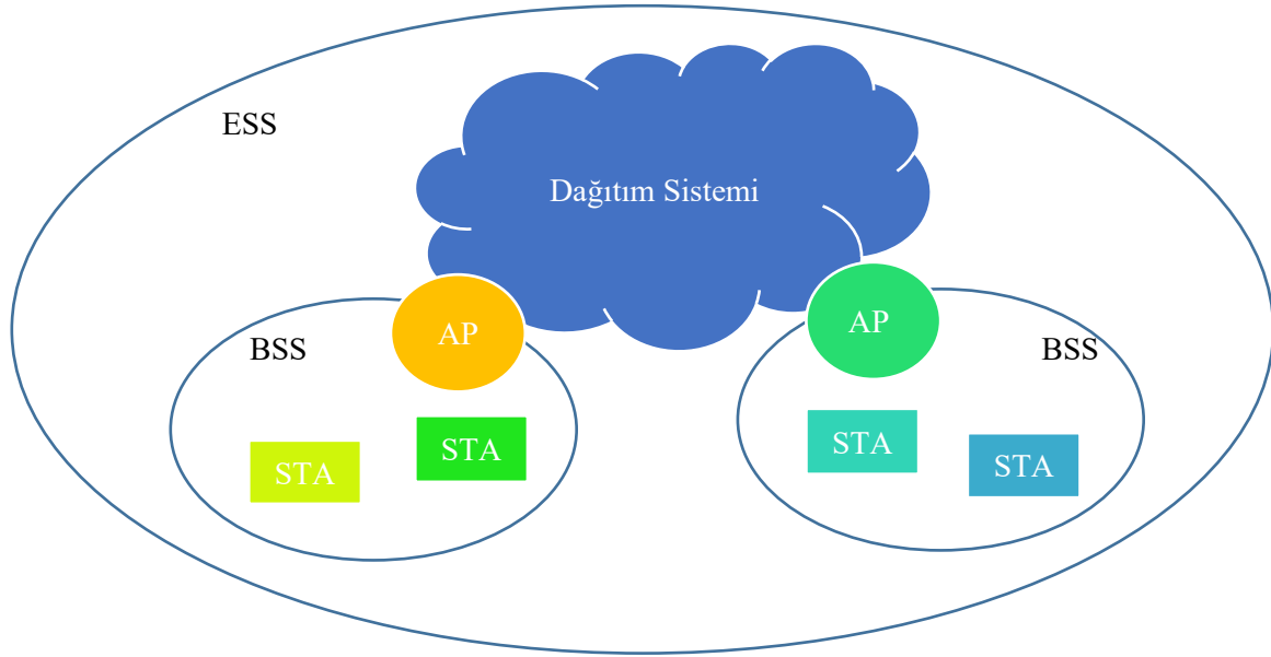
Şekil 27: Kablosuz Ağ Mimarisi
