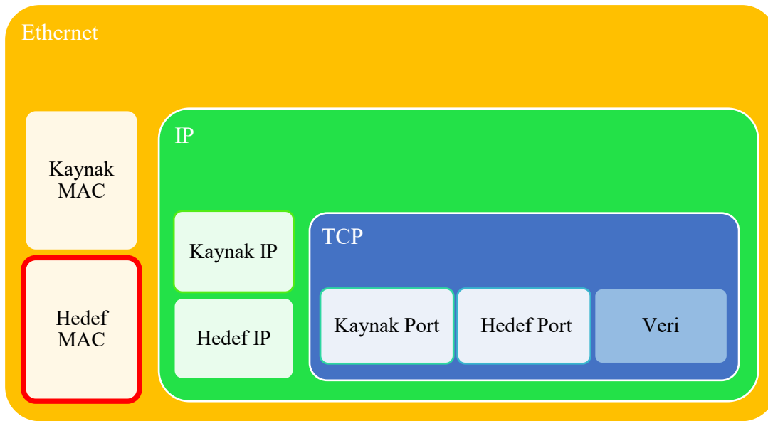
Şekil 26: Kapsülleme
