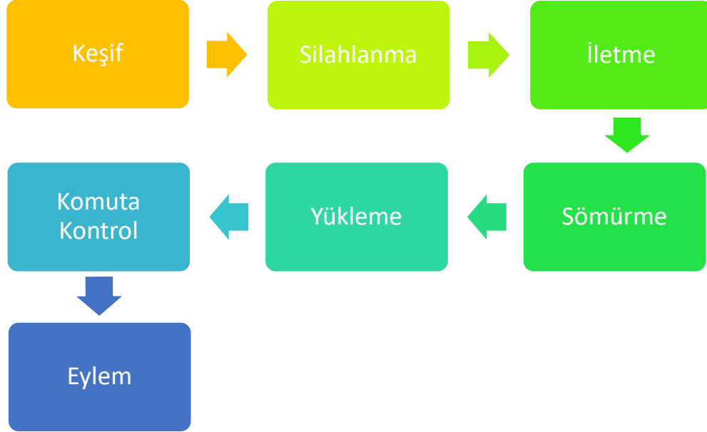
Şekil 31: Saldırı Aşamaları
