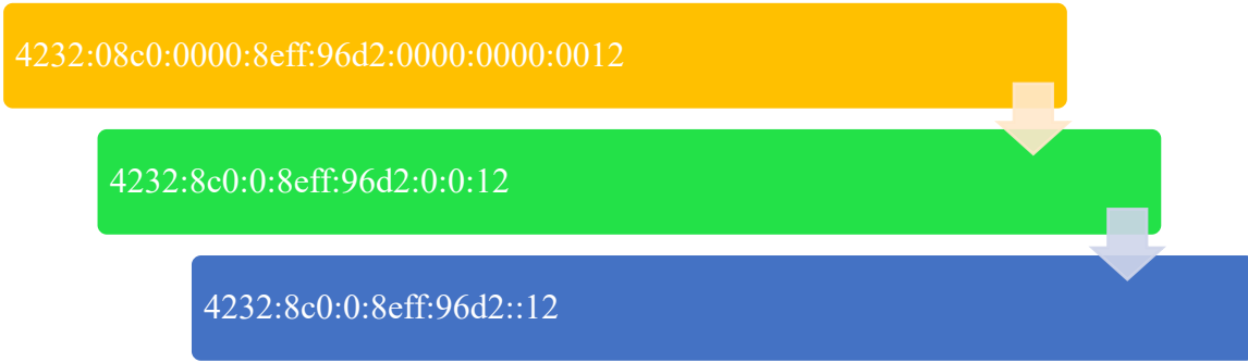
Şekil 24: IPv6 adresinin kısaltılması
