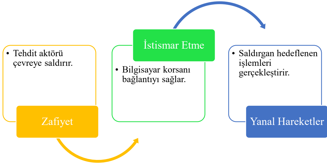
Şekil 32: Saldırı Zinciri
