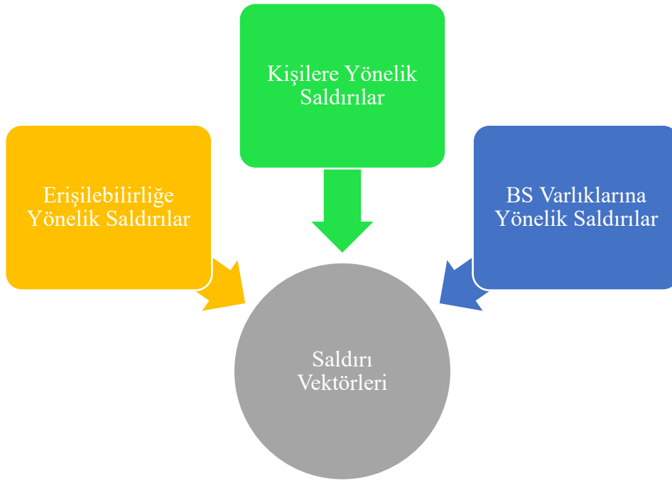
Şekil 34: Saldırı Vektörleri
