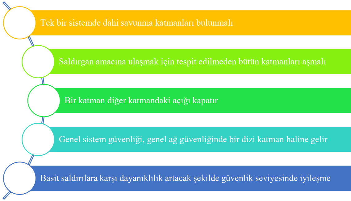
Şekil 35: Derinliğine savunma
