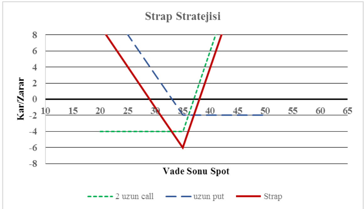
ŞEKİL 33: STRAP STRATEJİSİ
