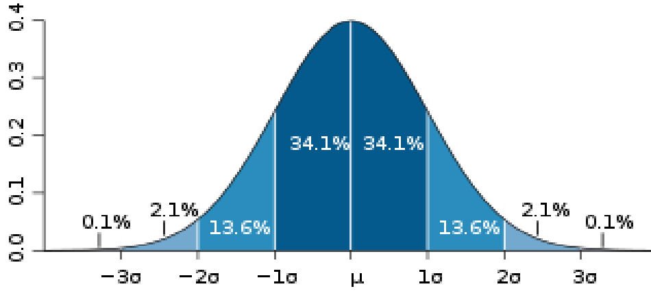
ŞEKİL 21: NORMAL DAĞILIM
