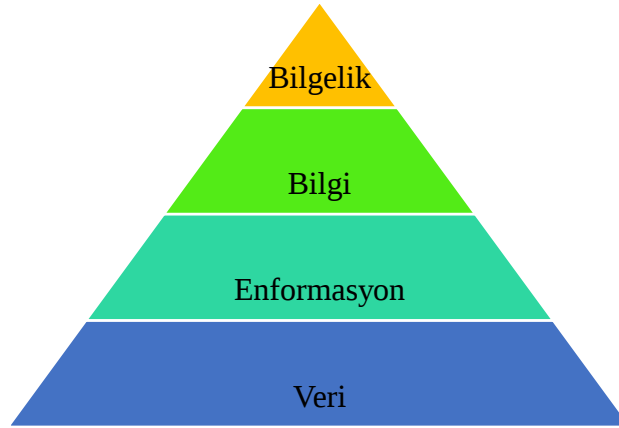
Şekil 43: DIKW Piramidi
