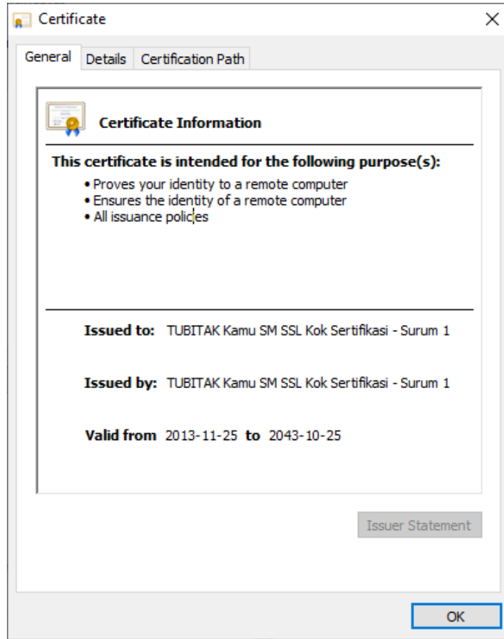
Şekil 52: Sertifika
