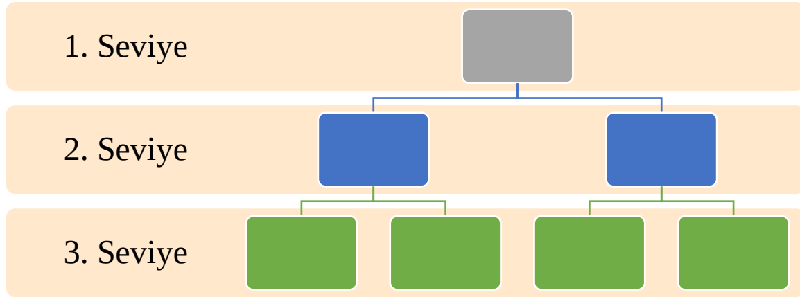
Şekil 8: Ağaç Topolojisi
