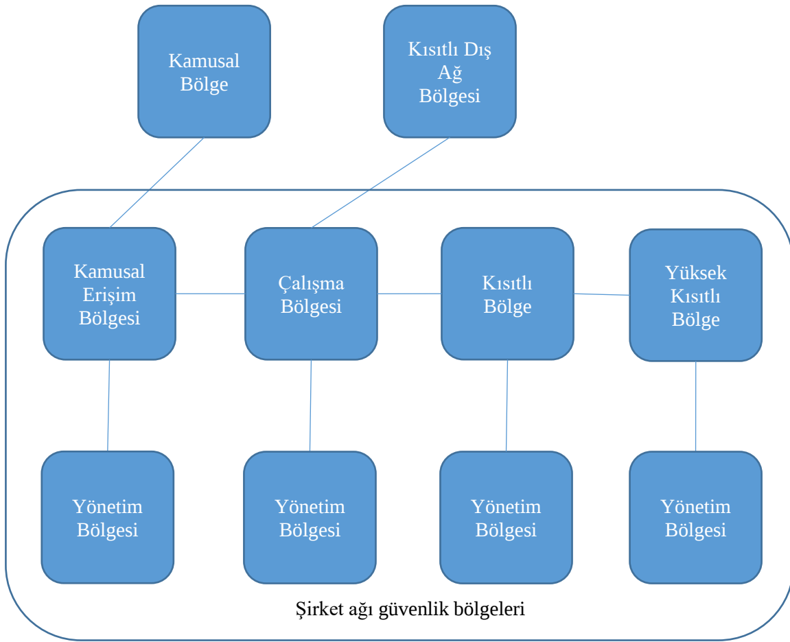
Şekil 35: Ağ güvenlik bölgeleri
