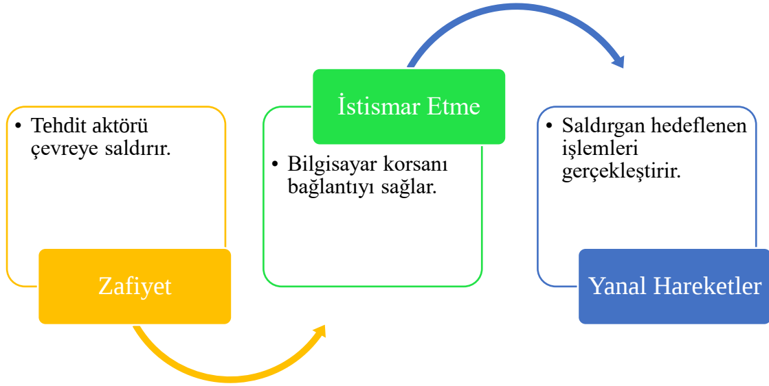
Şekil 31: Saldırı Zinciri
