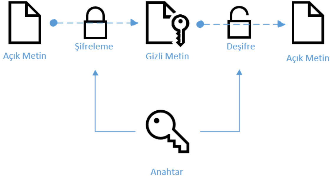
Şekil 48: Simetrik Şifreleme
