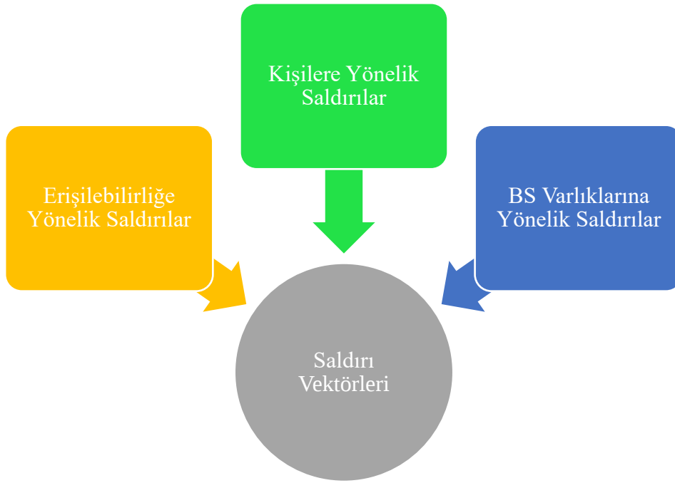
Şekil 33: Saldırı Vektörleri
