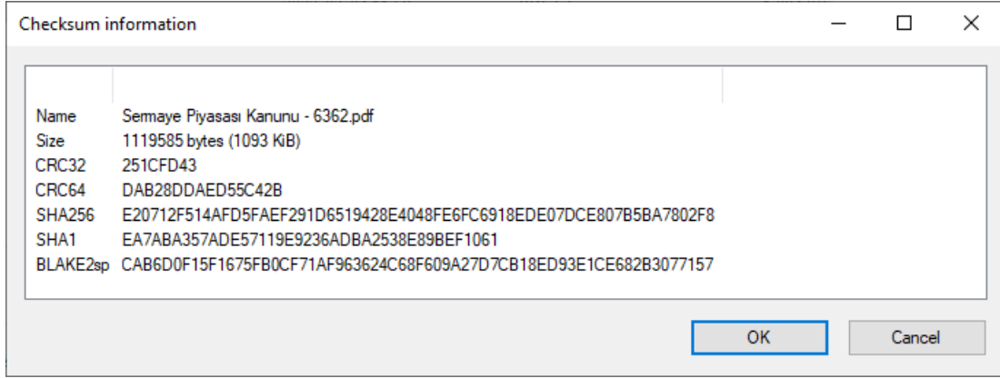
Şekil 47: Hash
